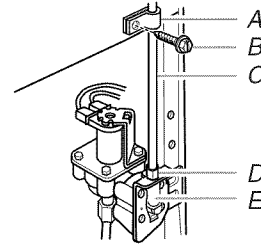
A. Abrazadera para tubería B. Tornillo de la abrazadera para tubería C. Tubería de cobre D. Tuerca de compresión E. Entrada de la válvula F. Válvula de cierre G. Tuerca de presión
