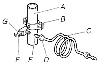
A. Tuyau de canalisation d'eau froide B. Bride de tuyau C. Tube en cuivre D. Écrou de compression E. Bague de compression F. Robinet d'arrêt G. Écrou de serrage
