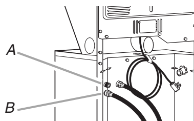
A. Valve du tuyau d'alimentation d'eau froide (haut) B. Valve du tuyau d'alimentation d'eau chaude (bas)
