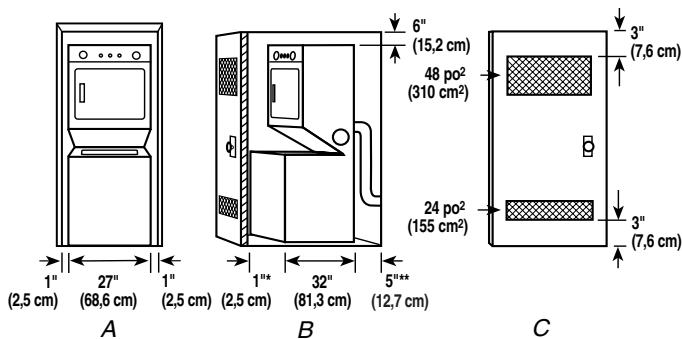
A. Encastrement
