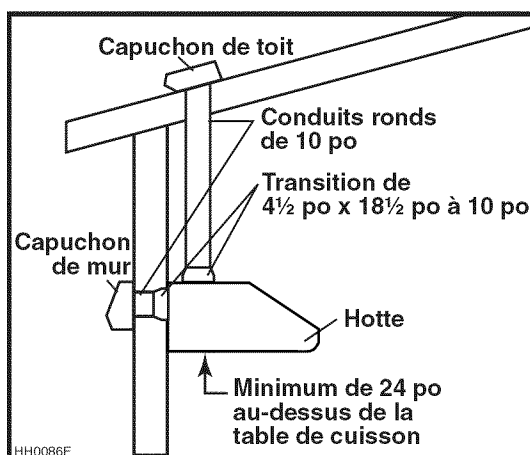
DEUX VENTILATEURS INTÉRIEURS CONDUITS TYPES
