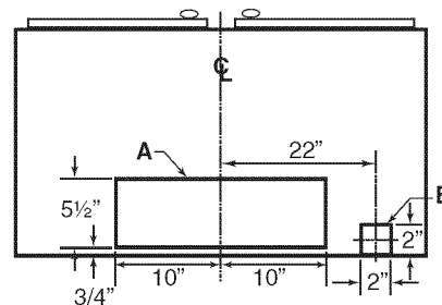
CAMPANA DE 48" CON DOS VENTILADORES INTERIORES
