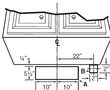
CAMPANA DE 48" CON DOS VENTILADORES INTERIORES
