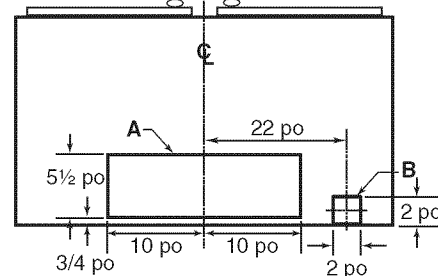
HOTTE DE 48 po À VENTILATEUR INTERNE DOUBLE
