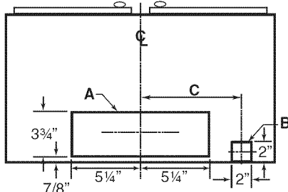
CAMPANA CON UN SOLO VENTILADOR INTERIOR
