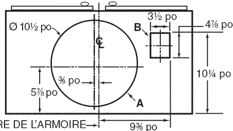
HOTTE AVEC VENTILATEUR EN LIGNE OU EXTÉRIEUR VUE DU DESSOUS DE L'ARMOIRE
