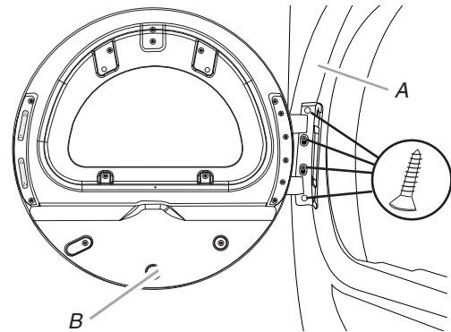
A. Panneau avant de la sécheuse B. Porte
