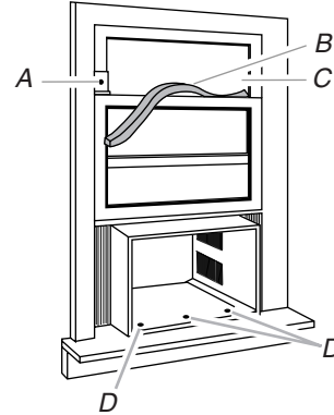
A. Soporte de seguridad de ventana B. Obturador de espuma del marco de la ventana C. Cristal de la ventana superior D. Tornillos Phillips de cabeza de cono achatado #10 x 1/2" (3)
