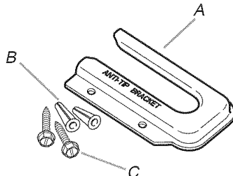
A. Bride antibascullement B. Chevilles de plastique (2) C. Vis n° 10 x \frac{1}{2} " (2)
