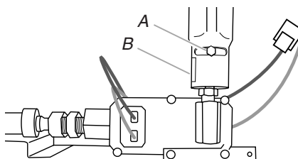
A. Vis de réglage de l'admission d'air
