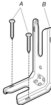
A. Vis n°12 x 1\frac{5}{8} " B. Bride antibascullement
