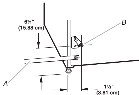
A. Canalisation d'arrivée de gaz NPT de \frac{1}{2} " B. Tuyau NPT de la sècheuse de \frac{3}{8} "
