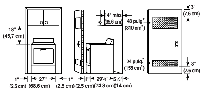
A. Lugar empotrado B. Vista lateral - clóset o lugar confinado C. Puerta del clóset con orificios de ventilación
