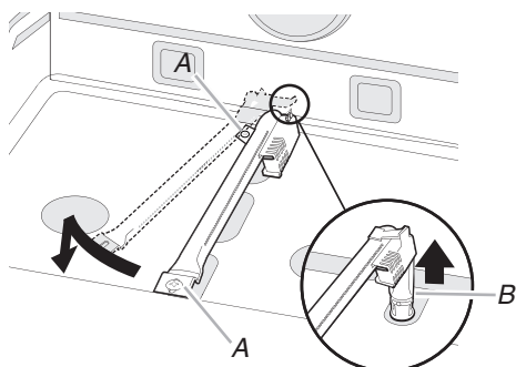
A. Vis du brûleur de cuisson au four B. Orifice du four
