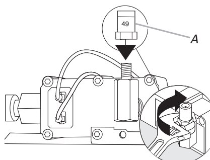
A. Gicleur du brûleur de cuisson au four au gaz naturel numéro 49
