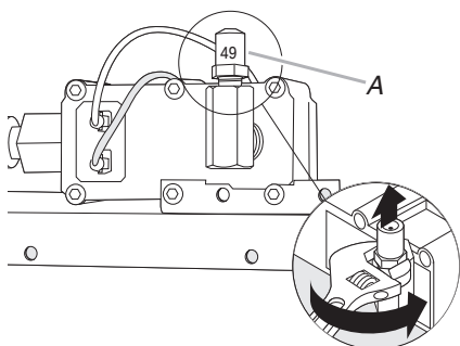
A. Gicleur du brûleur de cuisson au four au gaz naturel numéro 49
