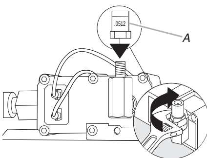
A. Gicleur noir au gaz propane numéro .0512
