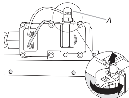
A. Gicleur du brûleur de cuisson au four au gaz propane numéro .0512
