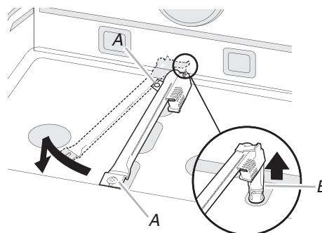
A. Vis du brûleur de cuisson au four B. Orifice du four
