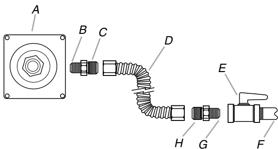
A. Détendeur B. Utiliser un composé d'étanchéité C. Raccord d'adaptation (avec filetage mâle NPT de 1/2") D. Raccord flexible E. Robinet d'arrêt manuel F. Tuyau de gaz de 1/2" ou 3/4" G. Utiliser un composé d'étanchéité H. Raccord d'adaptation
