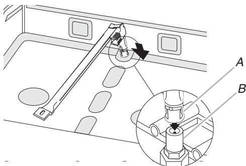
A. Brûleur de cuisson au four B. Gicleur du brûleur de cuisson au four
