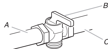
A. Canalisation de gaz B. Robinet d'arrêt (position de fermeture) C. Vers la cuisinière
